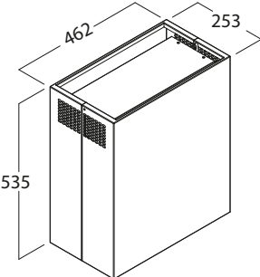
Camino filtrante Filtering chimney
