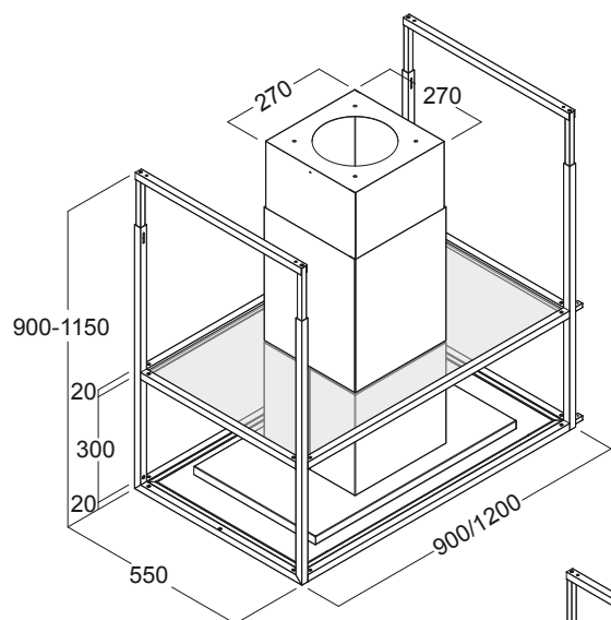
Cappa Hood
