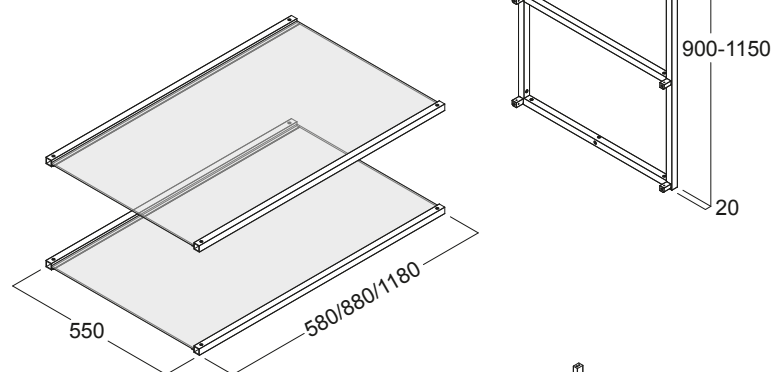
Mensola Shelf
