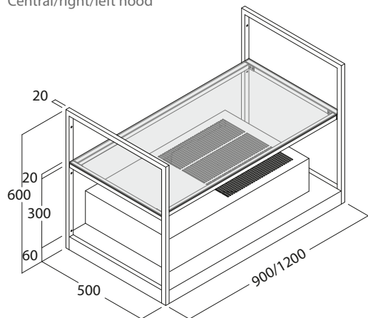
Mensola destra Right shelf
