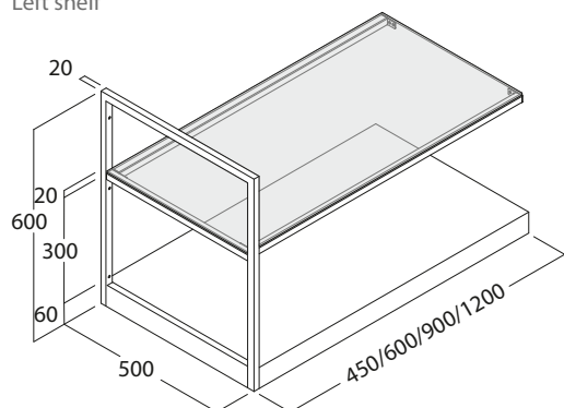
Mensola sinistra Left shelf
